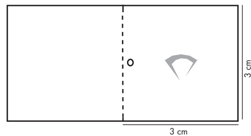
FUSTELLA N° 49 30 x 30 - doppio
